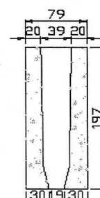
SECCIÓN A-A'
